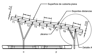
Frontal
