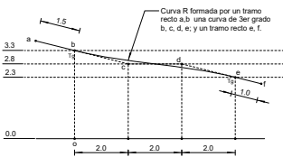
Esquema de curva R
