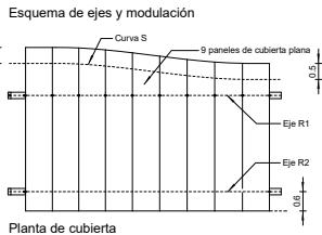
Planta de cubierta
