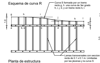
Planta de estructura
