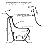
Sección Banca
