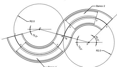
Planta
