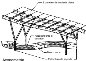
Axonometría
