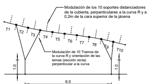
Esquema de ejes y modulación
