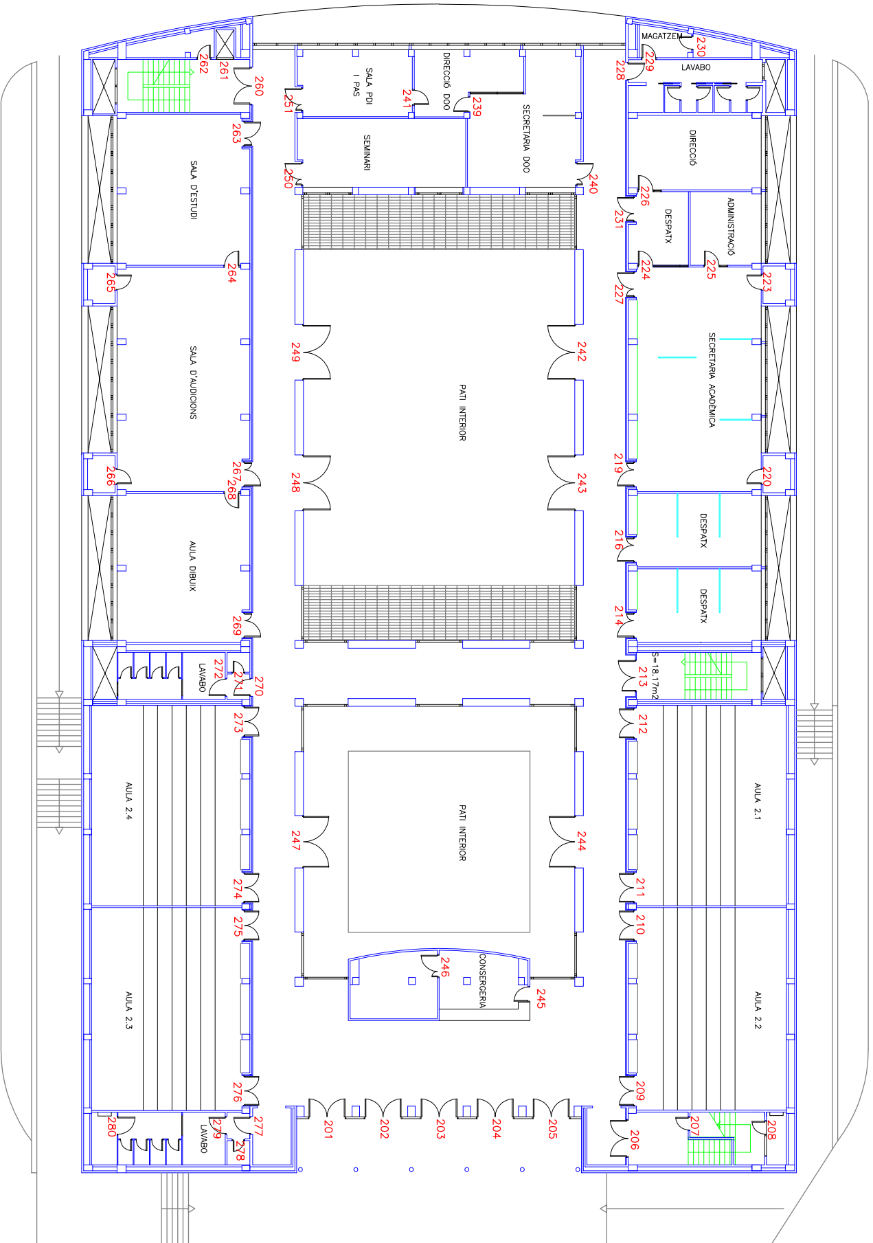
UNIVERSITAT POLITÈCNICA DE CATALUNYA EDIFICI TR8 – PLANTA 2
